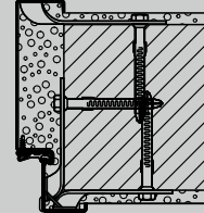
Köşe ve ilave kasa Dübel ankray montajı
