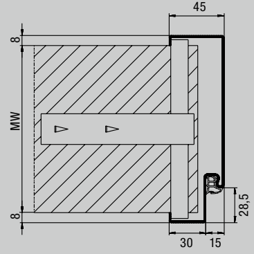
Profil 21101
