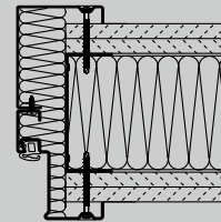
Köşe ve ilave kasa Vidalama montajı
