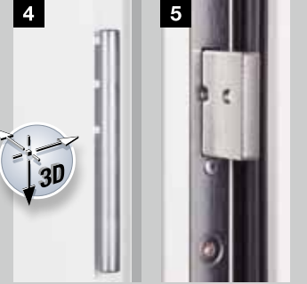
Kolay kapı ayarı için üç boyutlu ayarlanabilen makara şeritleri
