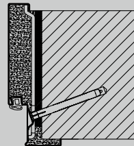
Tam kasa Duvar kalınlığı 175'e kadar çapraz sabitleme
