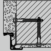
Dübel ankray montajı
