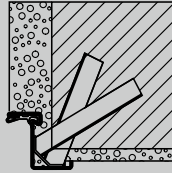
Duvar tuğla ankrayı ile montaj
